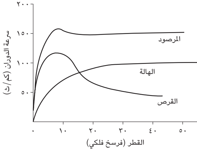
شكل ٦-٣: تمثيل تخطيطي لـ «منحنى الدوران» التقليدي الذي يُرى في أي مجرة قرصية.
