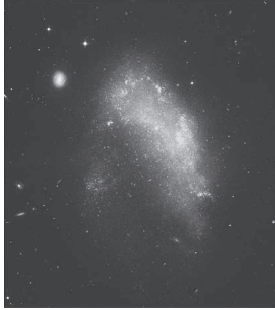
شكل ٥-٣: المجرة غير المنتظمة NGC 1427.
